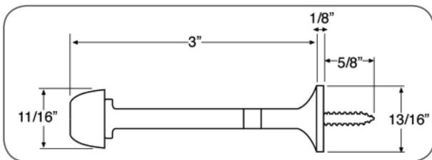
4679 - Door Stop
