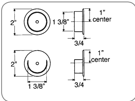
2820 - Pole Socket
